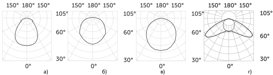
Рисунок 4: а) Микропризма поликарбонат 90°, б) Прозрачный поликарбонат, прозрачное закаленное стекло 120°, в) Опал 120°, г) Линза Ш2.
