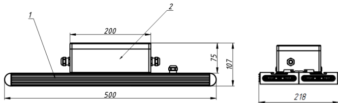
Рисунок 1 — Светильник Element БАП без системы крепления.
