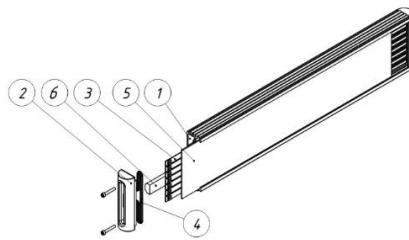
Рисунок 2 — Конструкция светильника Geniled Element.
