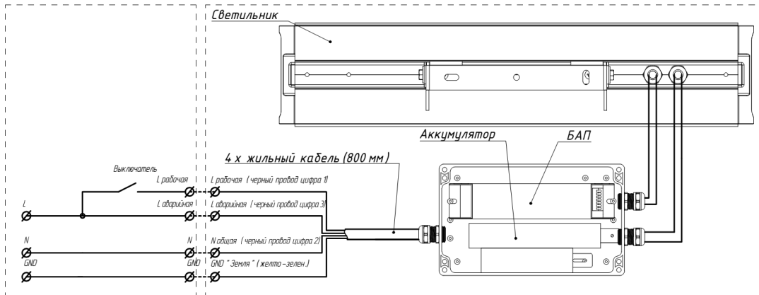
Рисунок 8 — Схема подключения аварийного светильника.
